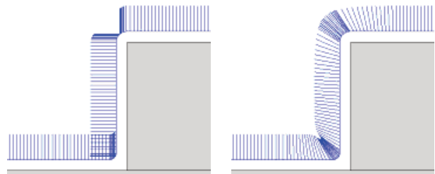
Fig. 7 Il est rare d'usiner une pièce avec l'outil strictement normal aux surfaces.
